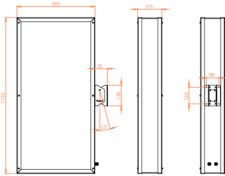
M01: Sıva üstü Montaj
