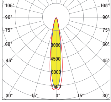
Polar Diyagram - 10°
